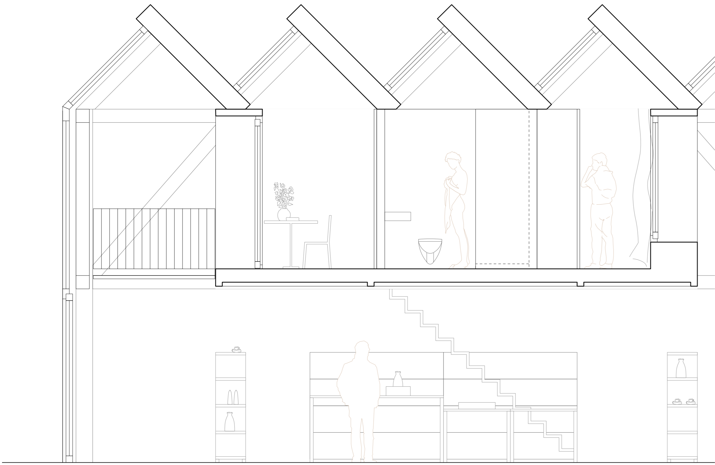
Schnitt
