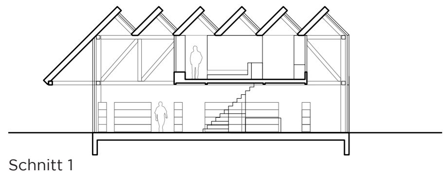
Schnitt 1
