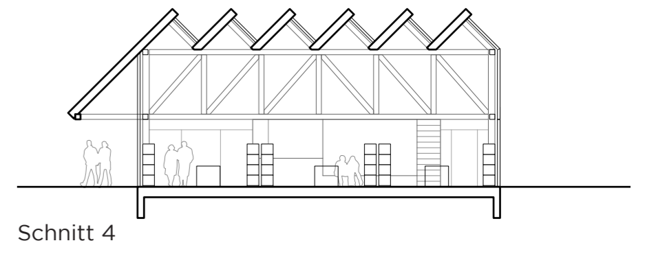
Schnitt 4
