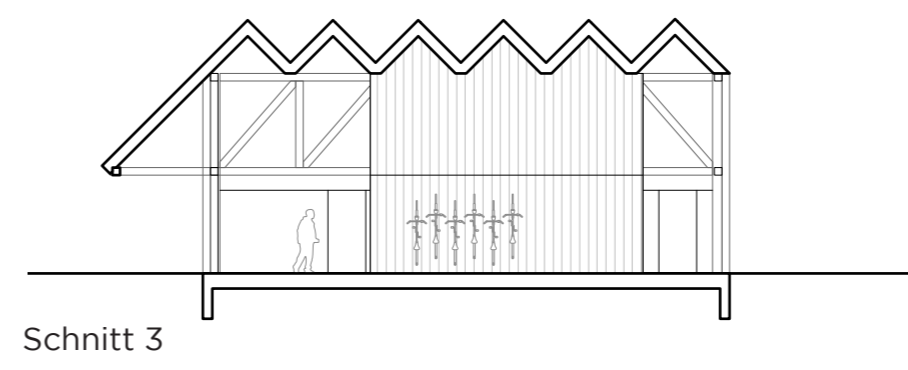
Schnitt 3
